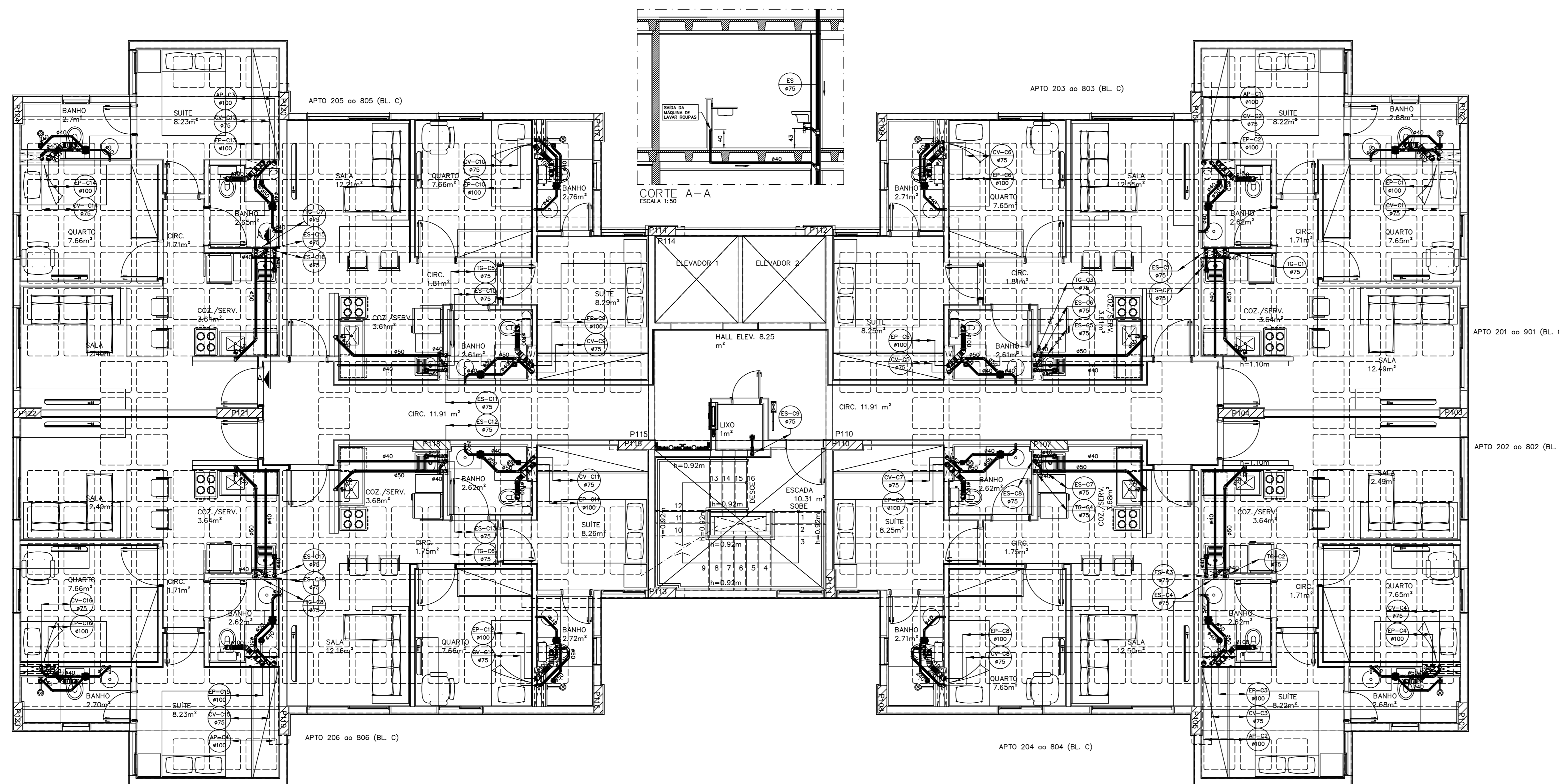
PLANTA BAIXA - 1° AO 8° PAVIMENTO-BLOCO C ESCALA 1:50
